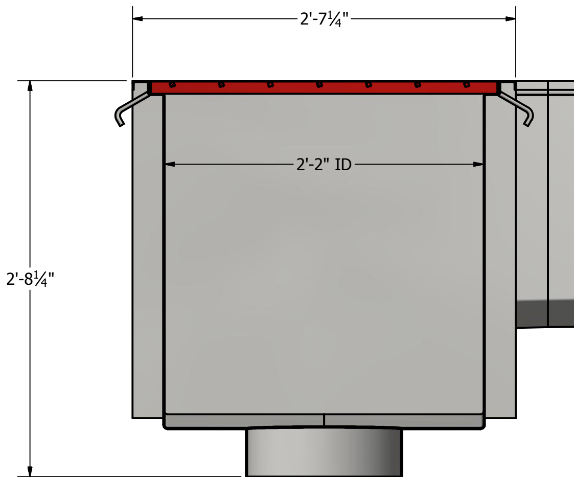
SECTION D-D
