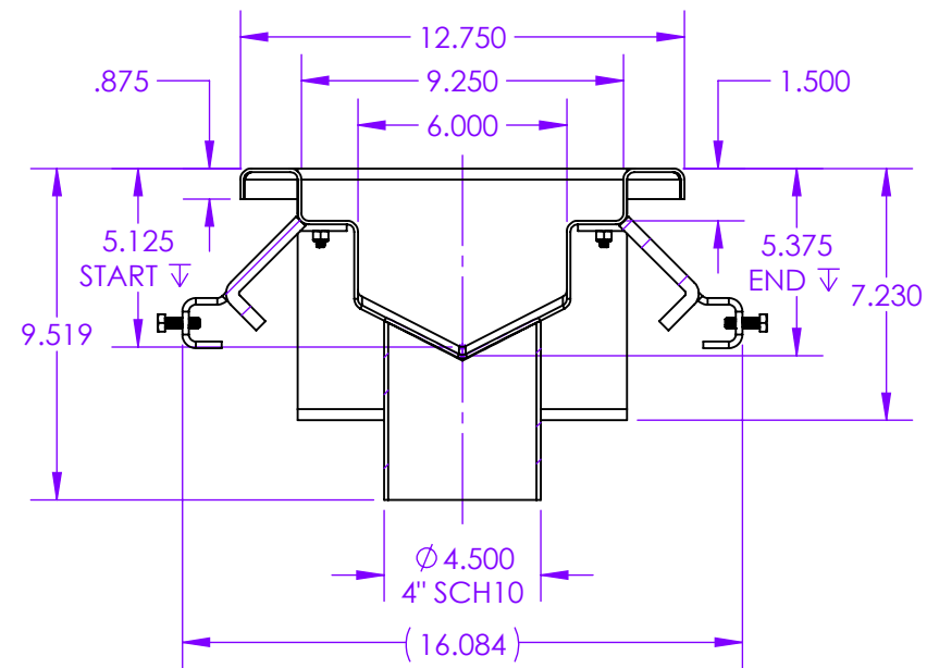
SECTION A-A SCALE 1 : 6
