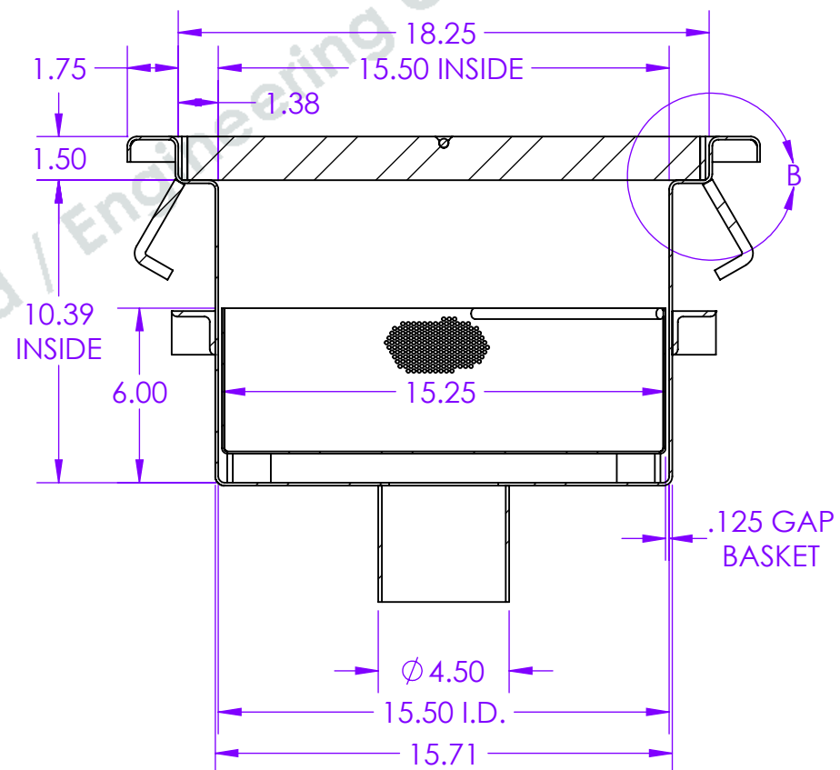
SECTION A-A SCALE 1 : 6
